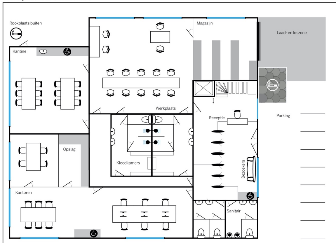
Figuur 6. Grondplan oorspronkelijke situatie
