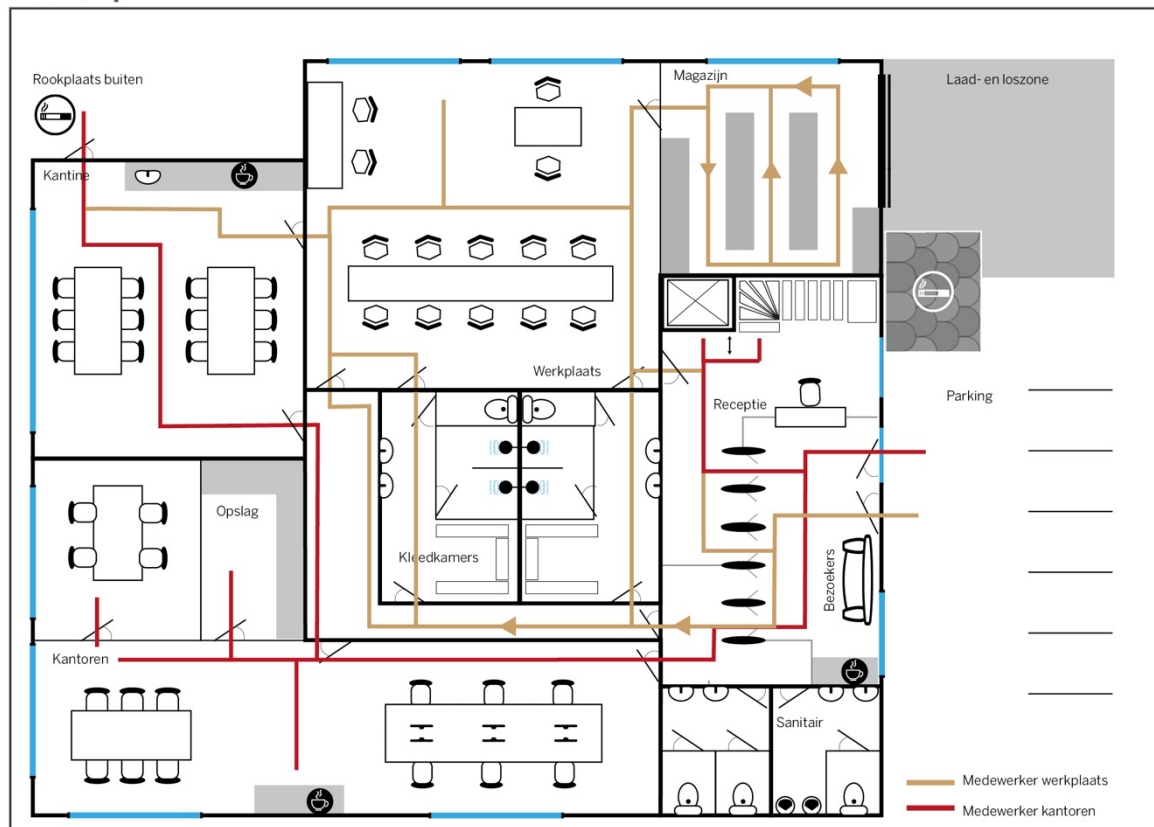
Figuur 11. Circulatieplan
